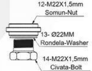
A-M22X1,5
